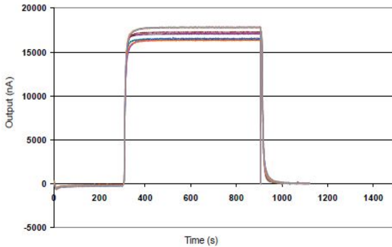
图6 H 2 S通道灵敏度温度特性
