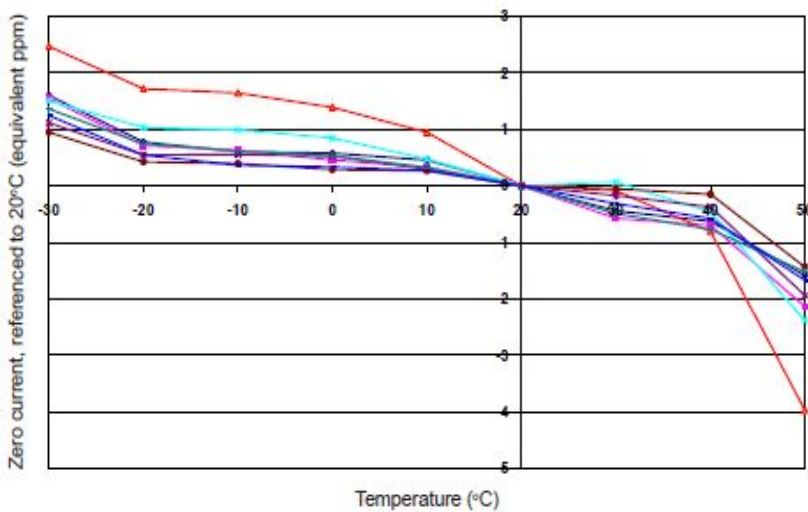
图2 CO通道零点温度特性
