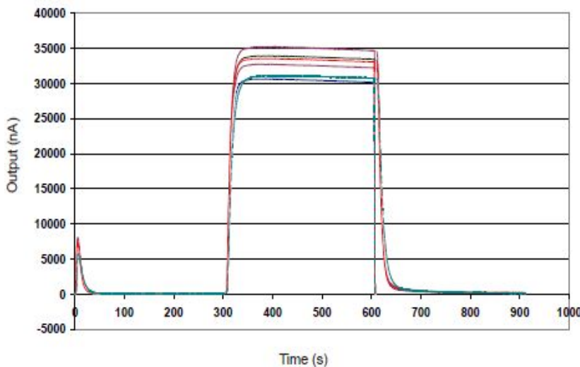
图3 CO通道对800ppmCO的反应
